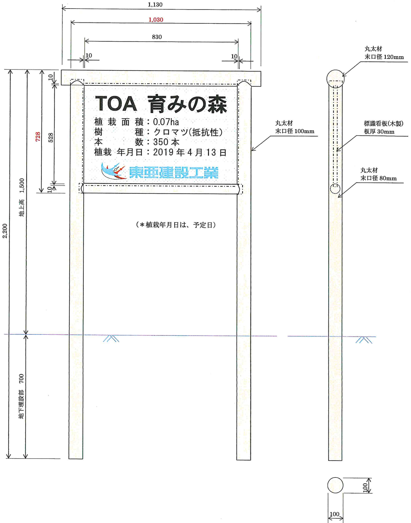
社会貢献の森 標識詳細図
