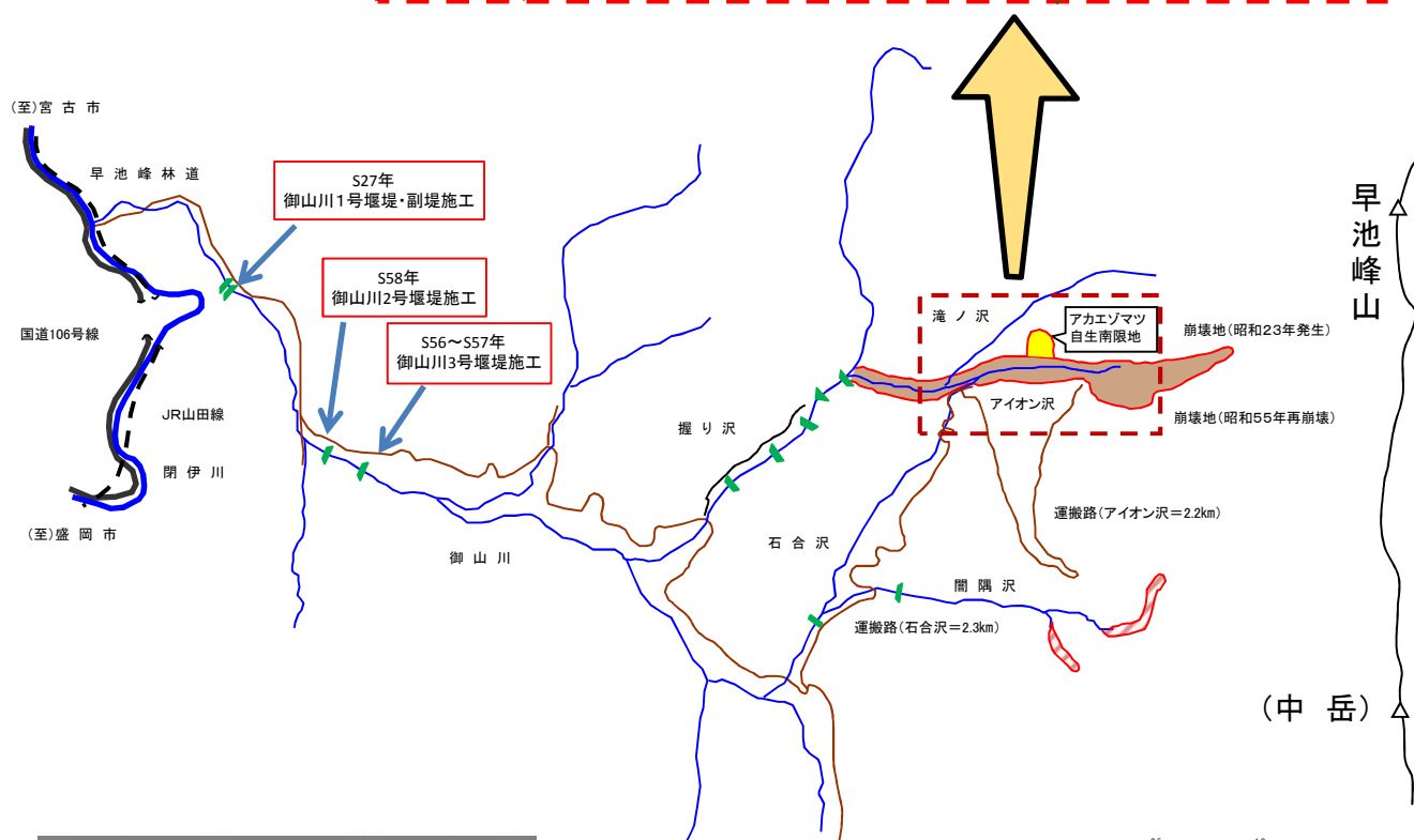
アイオン沢下流部の御山川1号堰堤
