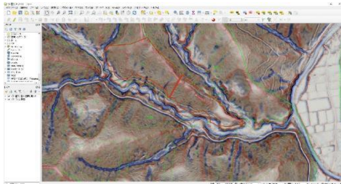
【QGISでCS立体図を表示】
