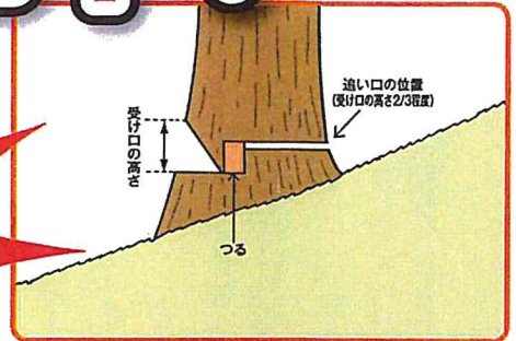
受け口を作る胸高直径 (40cm→20cmに拡大)
