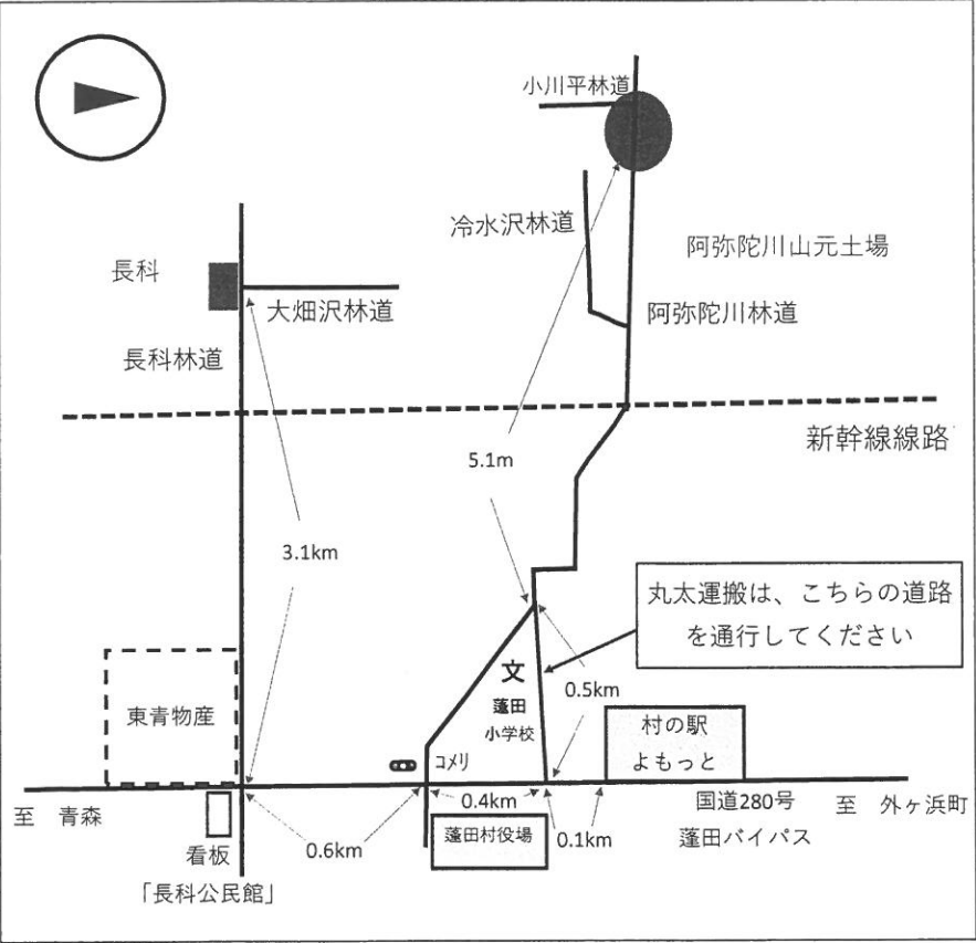
経路図
