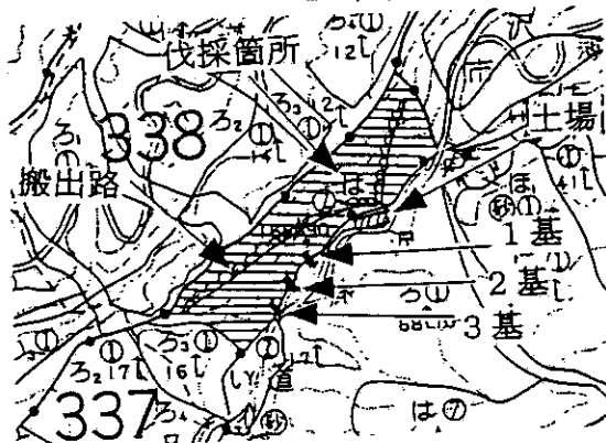
施工位置図（図-1）
