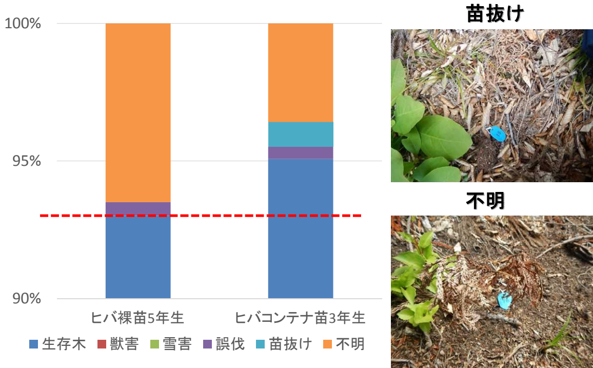
図-3 枯死原因
