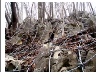
ロープ伏工完成(平成22年3月4日)
