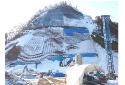
吹付砕工施工状況(平成22年1月22日)
