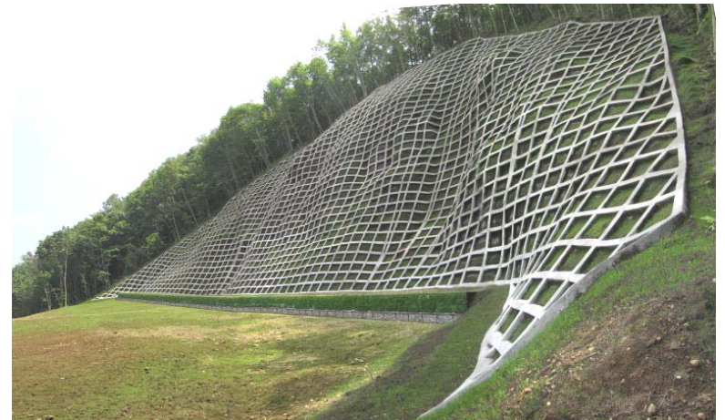
吹付枠工 工事完成 (平成21年8月4日)
