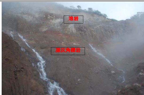
⑦地すべり性崩壊の滑落崖・溶岩下面から大量の湧水が生じる
