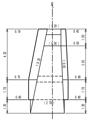
右岸側面図
