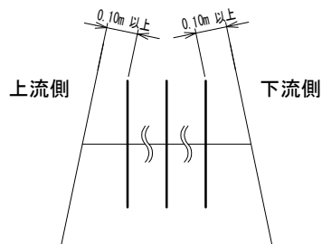
配置側面図
