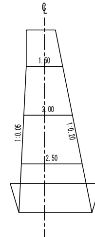
断面図
