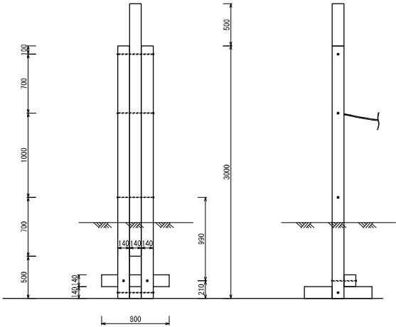
側面図
