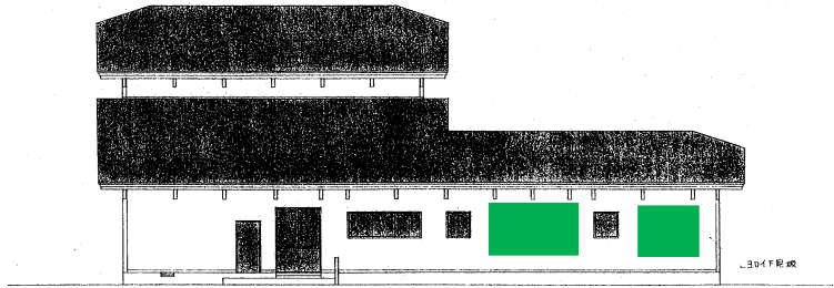
西立面図
