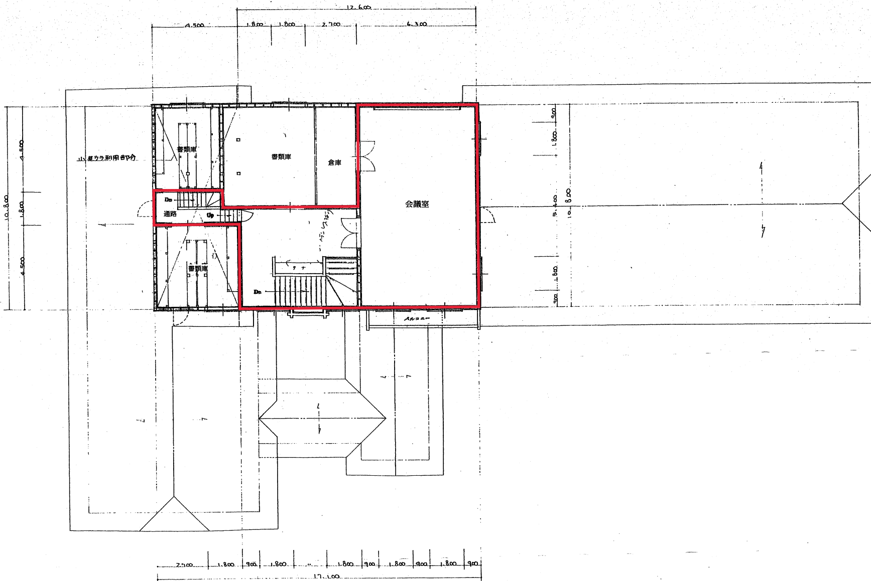
2 階 平 面 図
