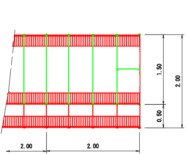
平面図
