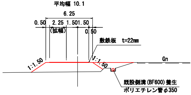
起点拡幅部(A-A断面)
