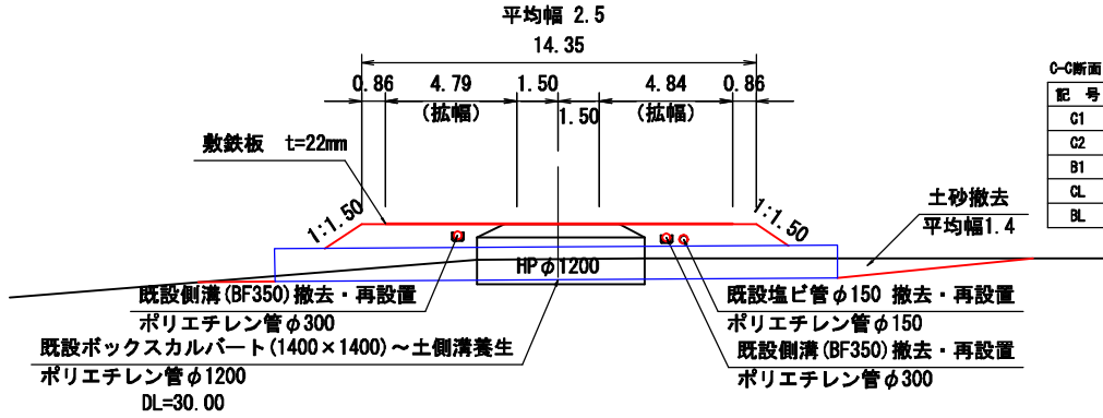
既設暗渠管横断面(C-C断面)
