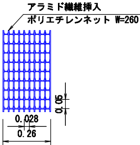
中間固定ピン
