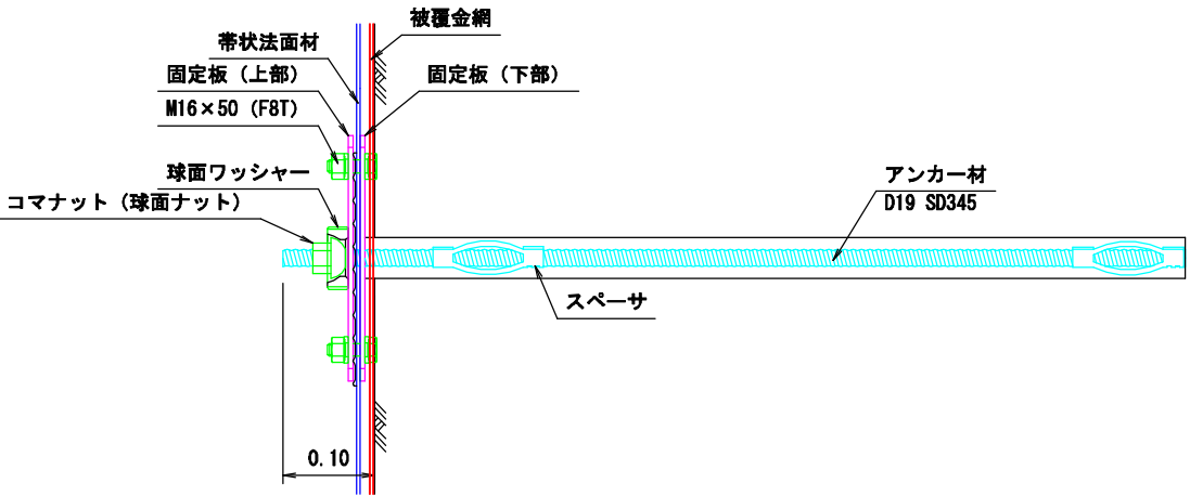
構造概要図
