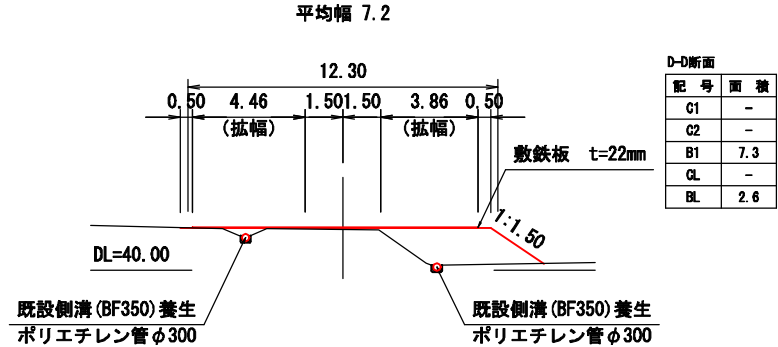
盛土部(D-D断面)
