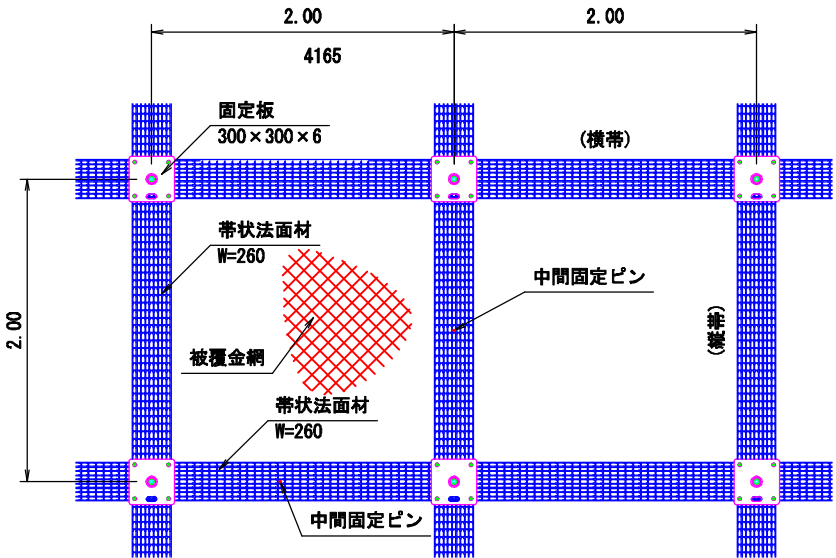
固定板詳細図
