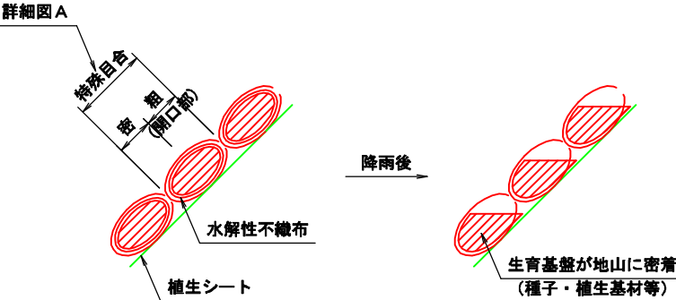
詳細図 A
