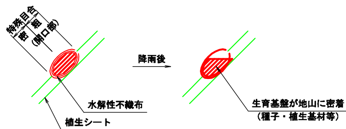
詳細図A
