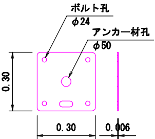
固定板詳細図
