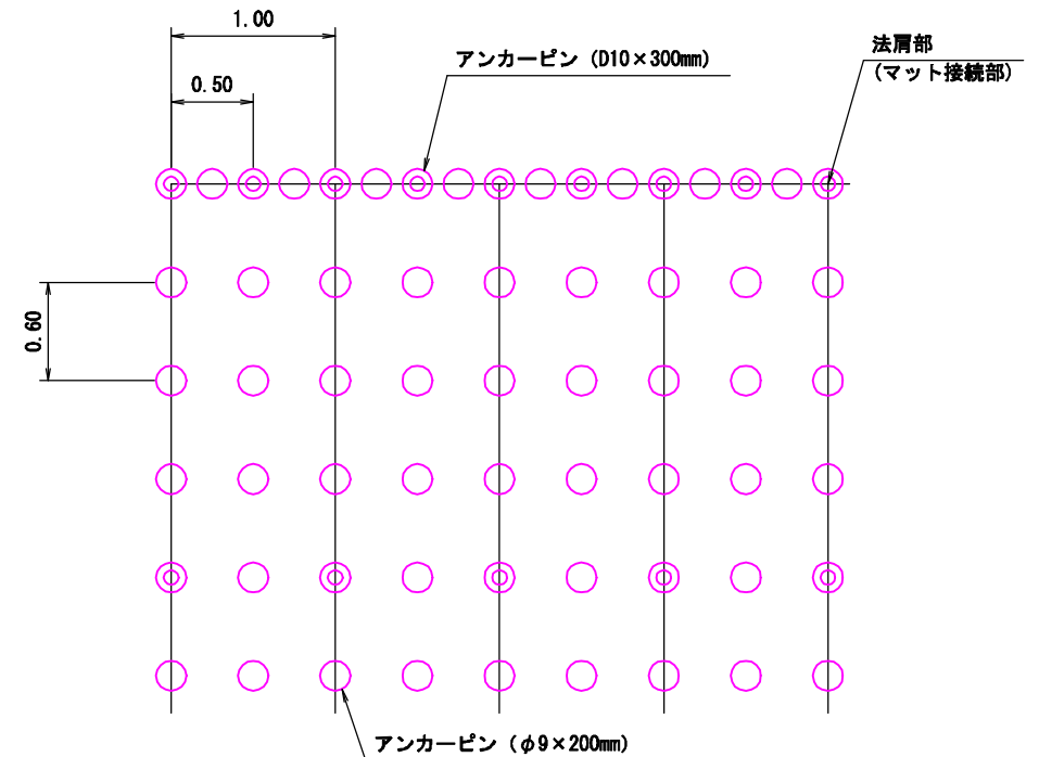
平面図
