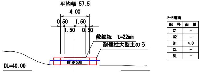
暗渠管横断面(E-E断面)
