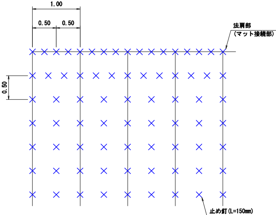
平面図
