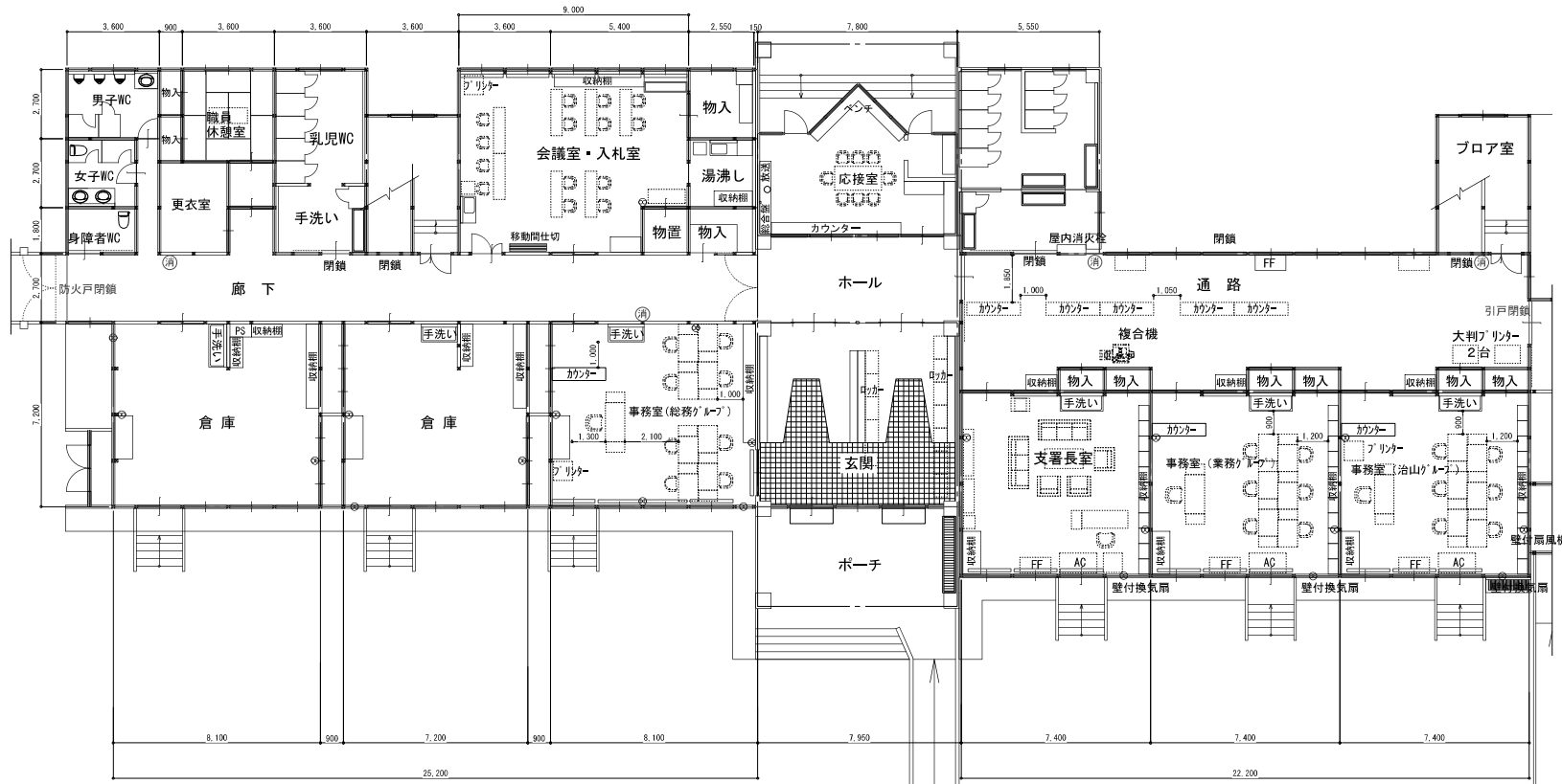
飯庁舎平面図 S=1/150
