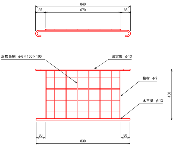
端部枠
