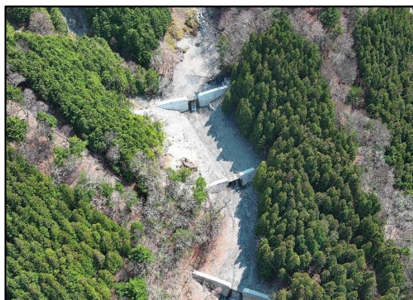
谷止工 (三好市東祖谷 三嶺国有林)
