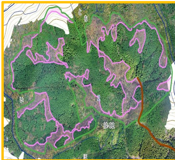
オルソ画像による最新の林況確認 谷相山国有林
