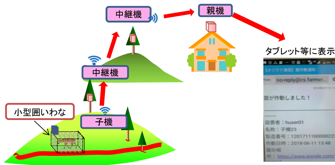
簡易無線通信を活用したシカのわな遠隔捕獲通知システム
