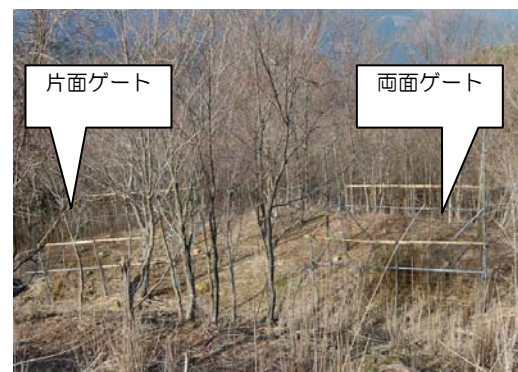
写真 4 足場用パイプを用いた囲いわな
