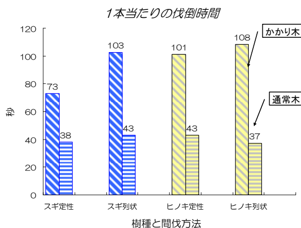
図 2 かかり木と通常木の伐倒時間の比較 (樹種別・間伐方法別)
