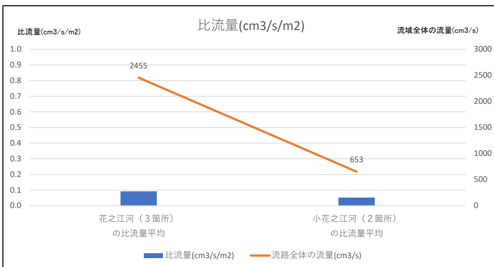
図表 4-7 比流量、2回目計測 (R元年10月1日)
