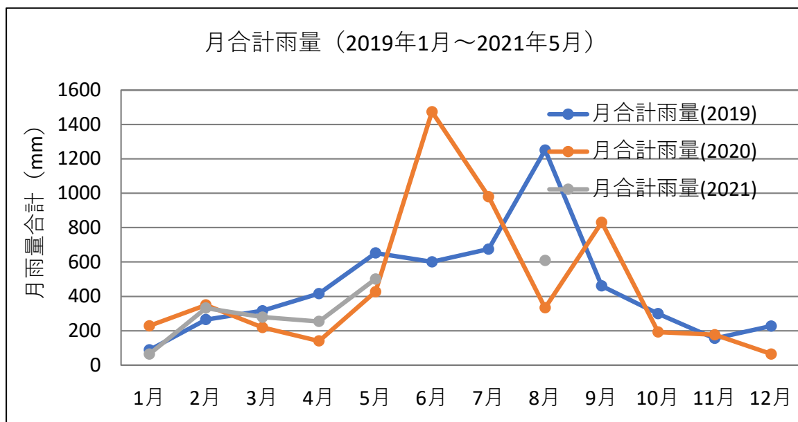
図表 4-19 黒味岳の月別合計雨量（2019/1/1～2021/5/21）
