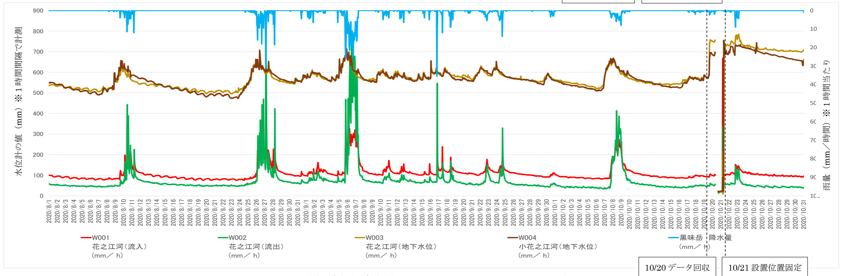
図 4-2 水位と降水量の変動 (上 2020 年 5 月～7 月、下 2020 年 8 月～10 月)
