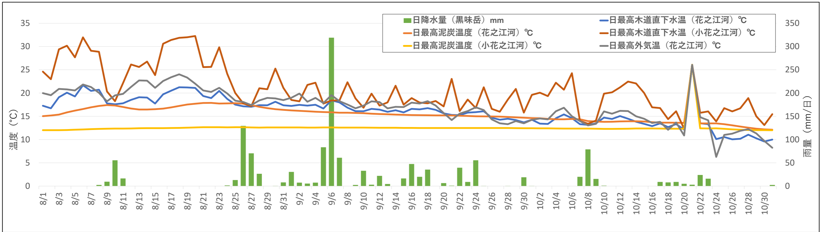
図 4-16 温度と降水量の変動 (上 2020 年 5 月～7 月、下 2020 年 8 月～10 月)
