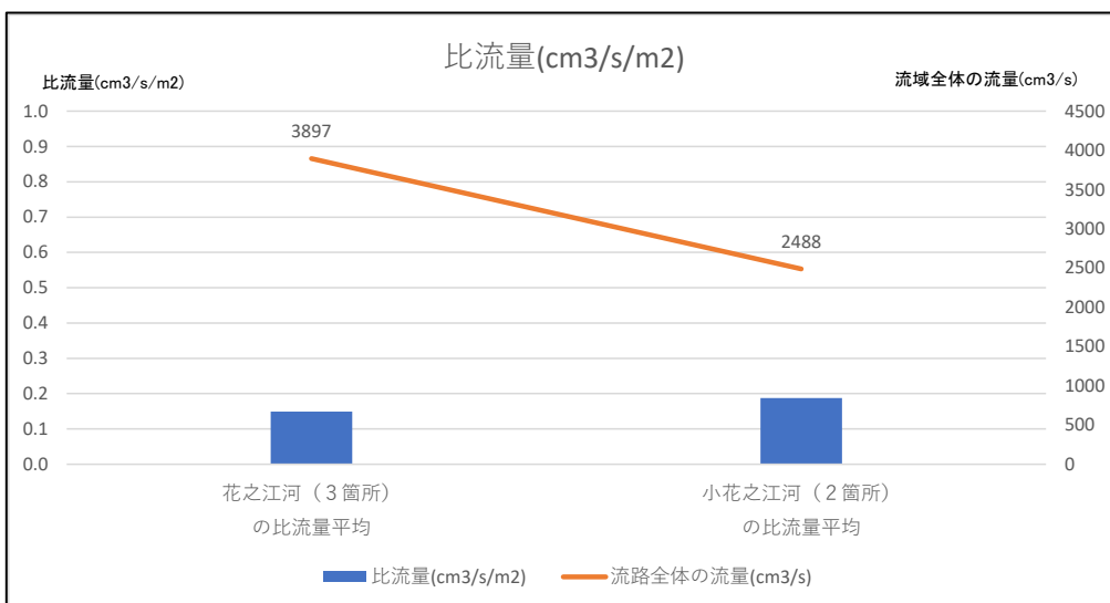
図表 4-12 比流量、7回目 (R2年10月20日)
