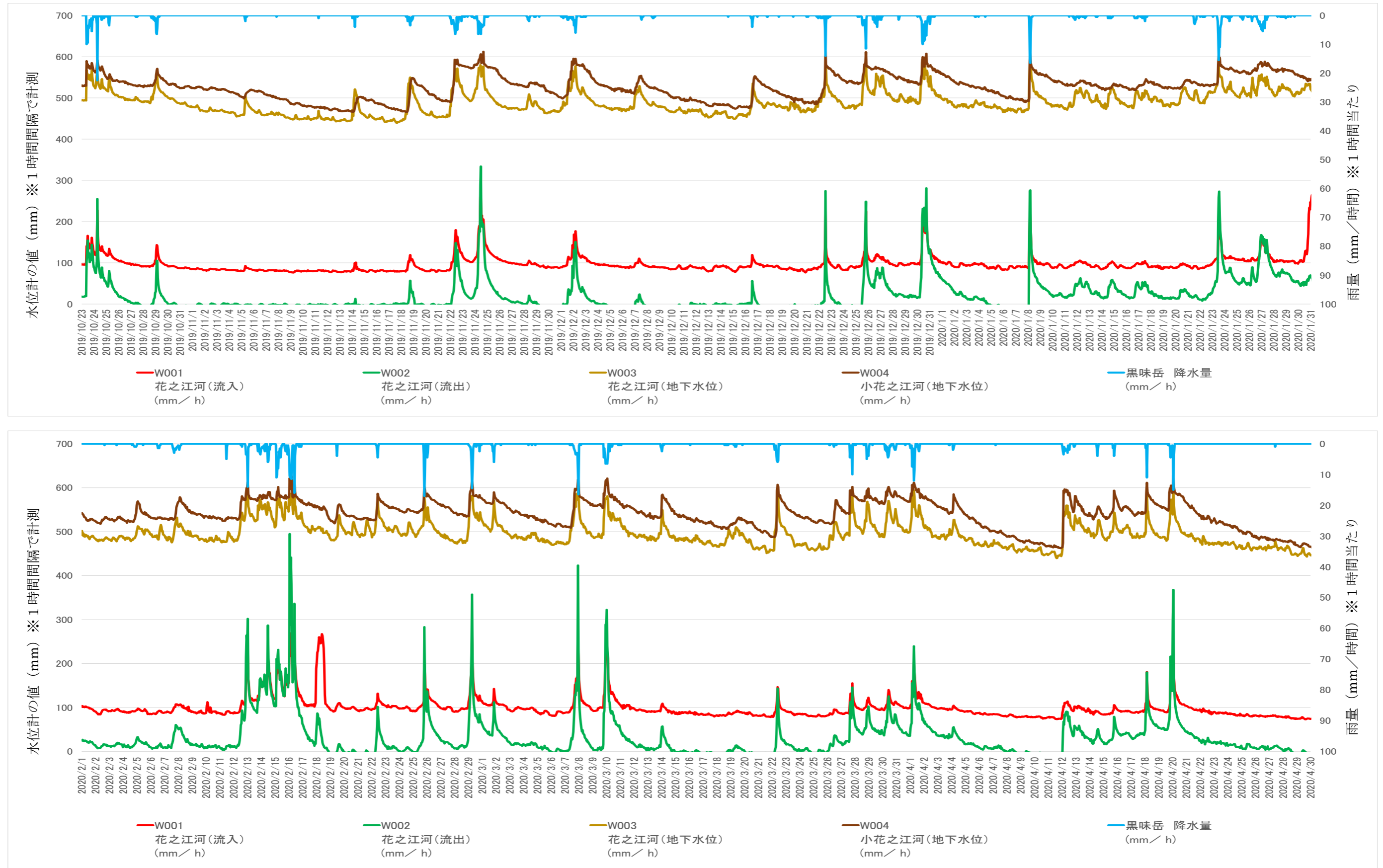
図 4-1 水位と降水量の変動 (上 2019 年 10 月～2020 年 1 月、2020 年 2 月～4 月)
