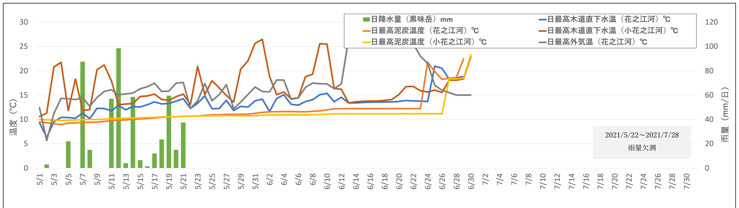
図 4-18 温度と降水量の変動 (2021 年 5 月～6 月)
