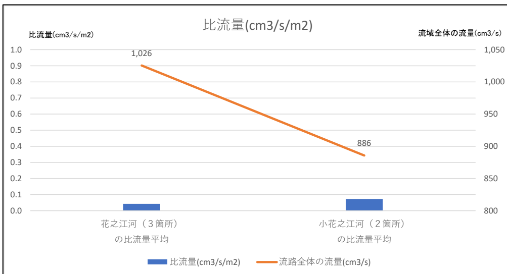
図表 4-9 比流量、4回目 (R元年12月10日)
