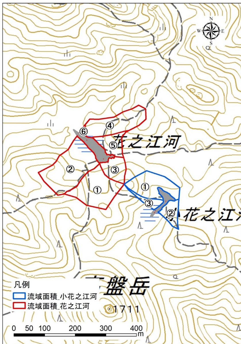
図 4-5 流域面積
