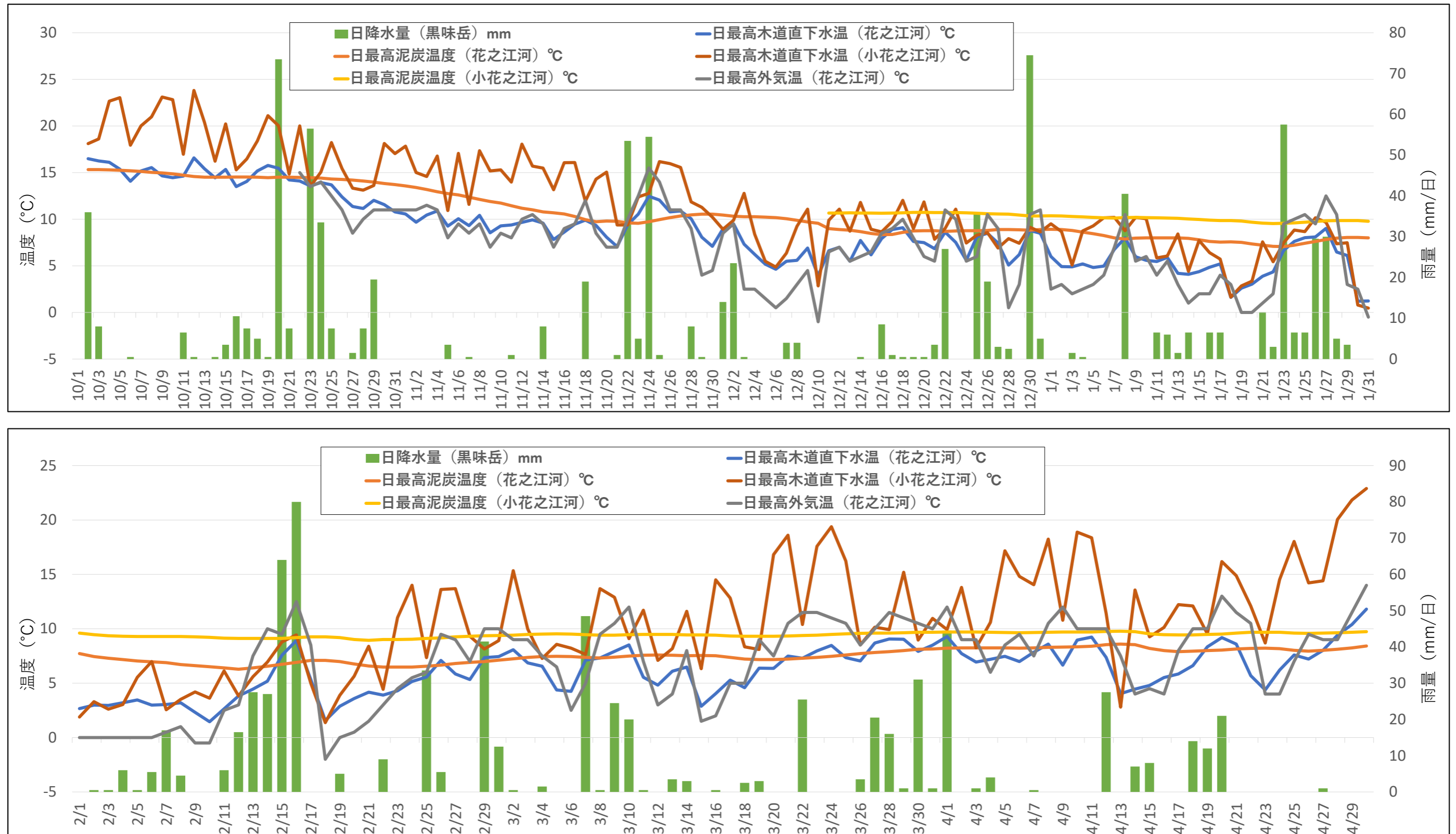
図 4-15 温度と降水量の変動 (上 2019 年 10 月～2020 年 1 月、下 2020 年 2 月～4 月)
