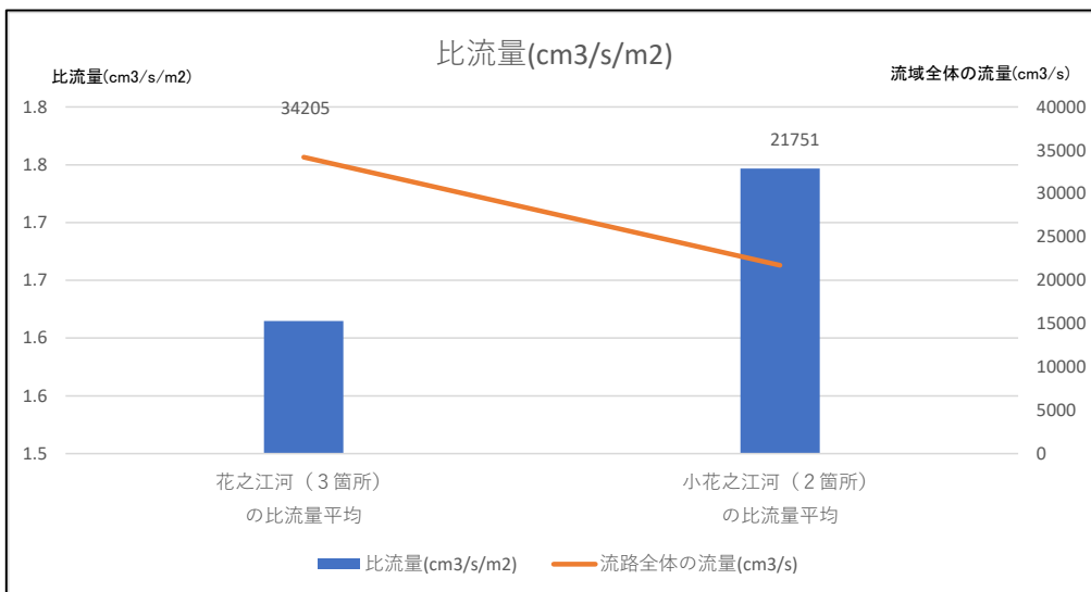
図表 4-11 比流量、6回目 (R2年9月17日)
