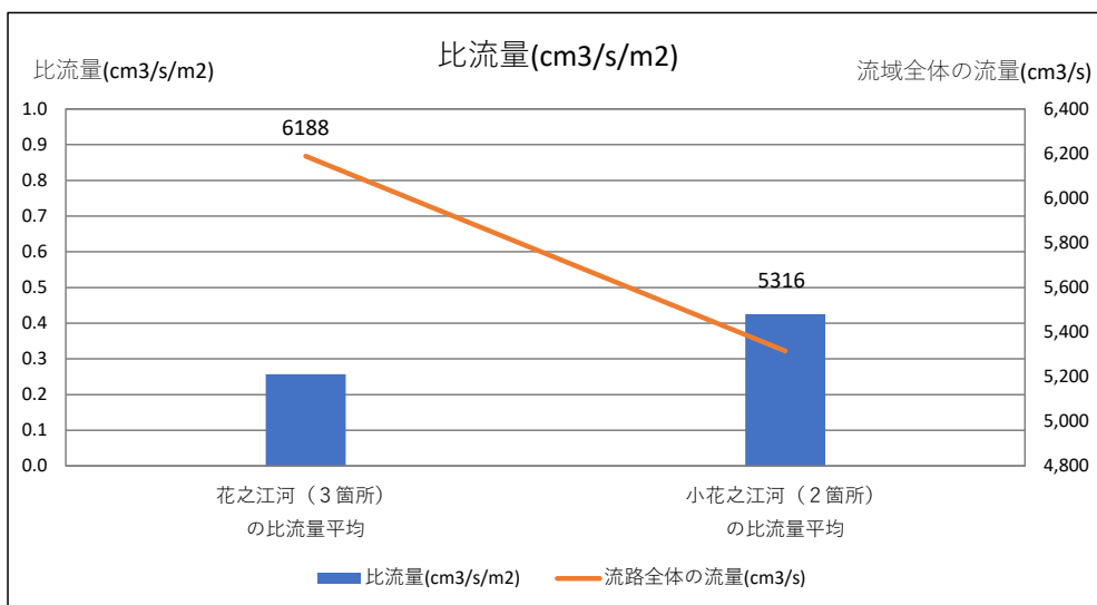
図表 4-13 比流量、8回目 (R3年6月13日)
