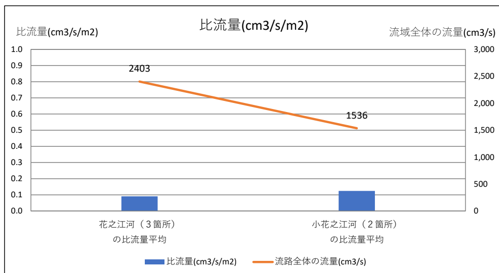
図表 4-14 比流量、9回目 (R3年9月20日)
