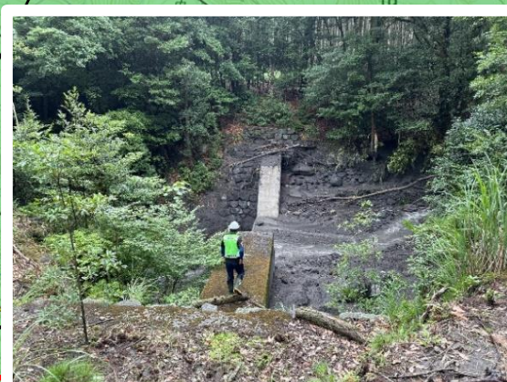
② 既設治山ダムの状況 治山ダムの背面が満杯となっている状況を確認
