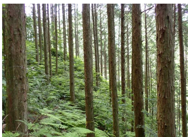
ヒノキ
