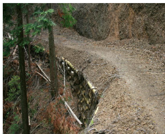
間伐に必要な丸太組を利用した低コスト路網
