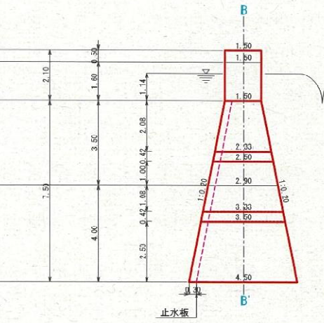
A~A' 断面图
