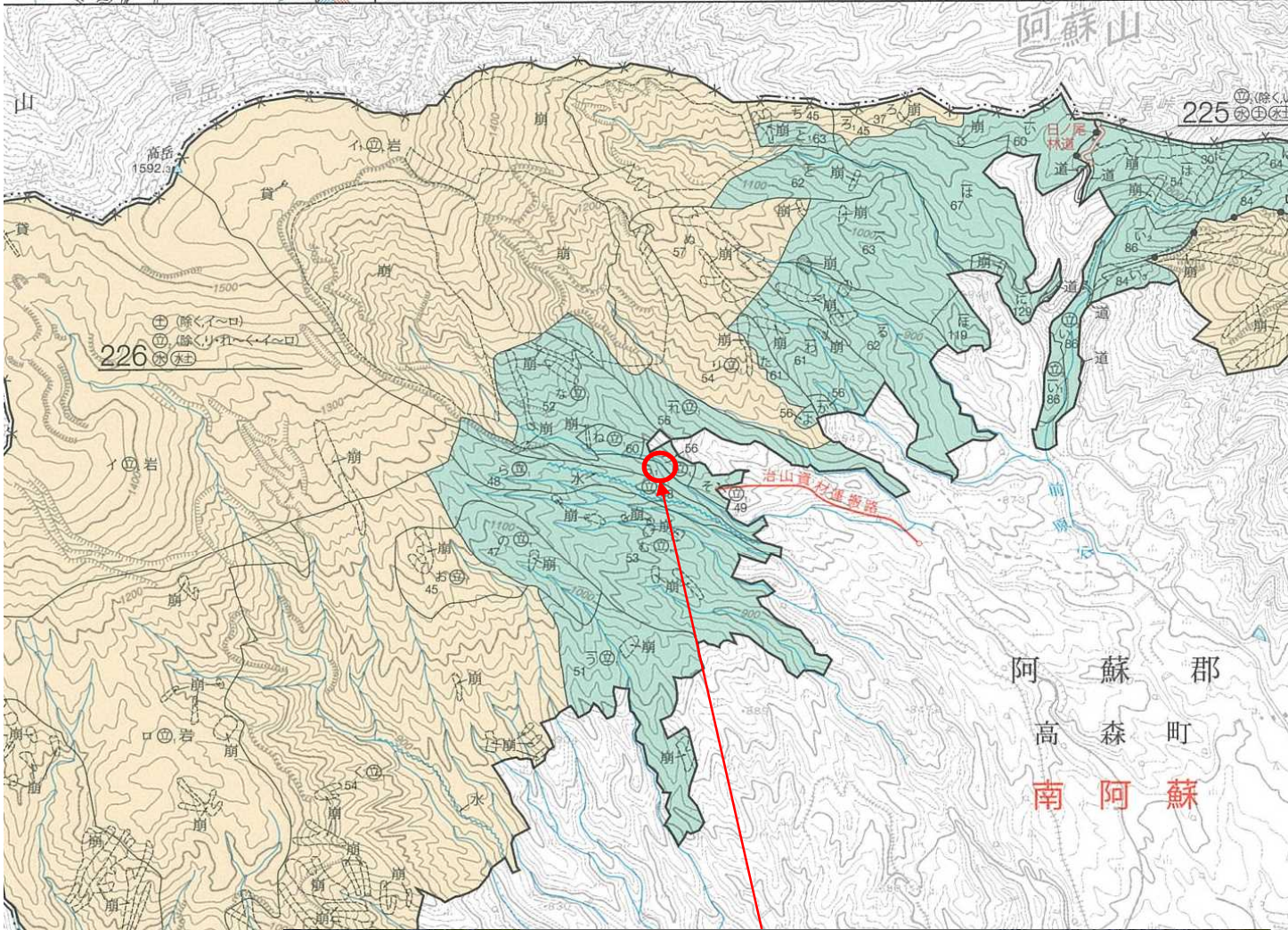
阿蘇岳治山工事
