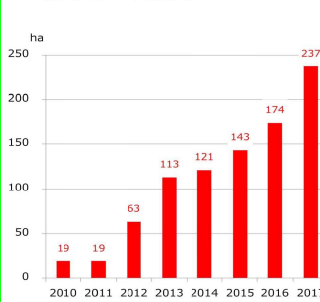
図-3 九州局における一貫作業システム（誘導伐）の実施状況
