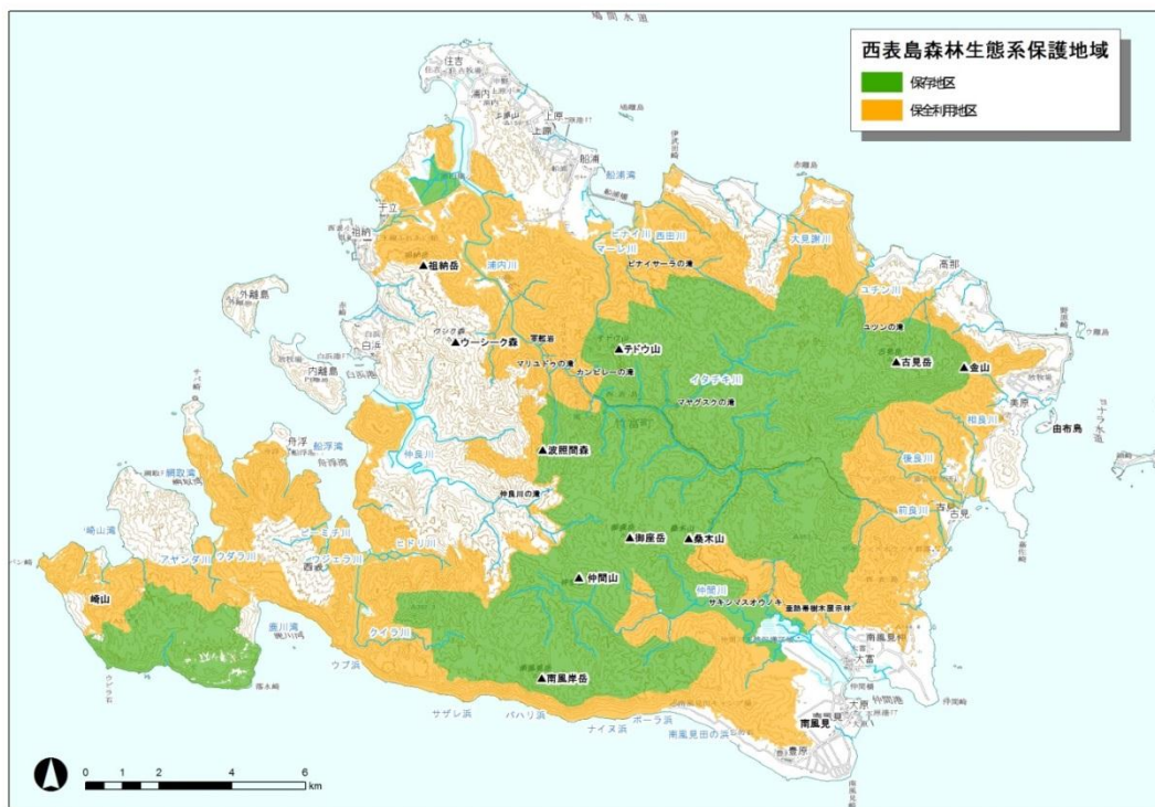
図1 西表島森林生態系保護地域位置図
