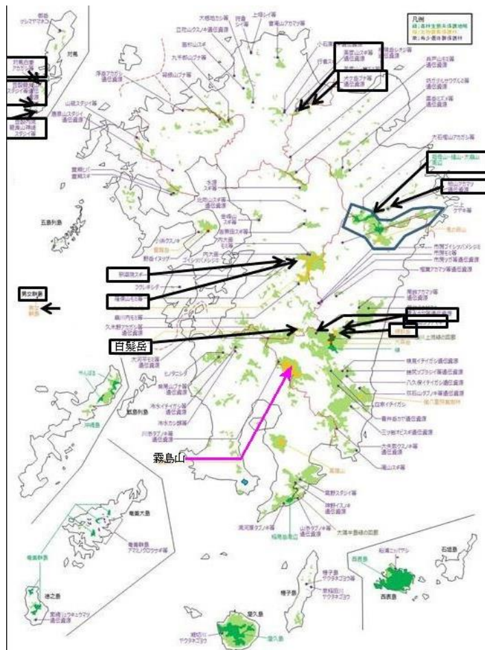
図1. 左図は九州管内の92箇所の保護林の位置を示す。四角枠は2018年度にモニタリングした保護林。視察した霧島山生物群集保護林と白髪岳生物群集保護林はゴシック文字で示した。霧島山生物群集保護林は2019年度のモニタリング予定地。
