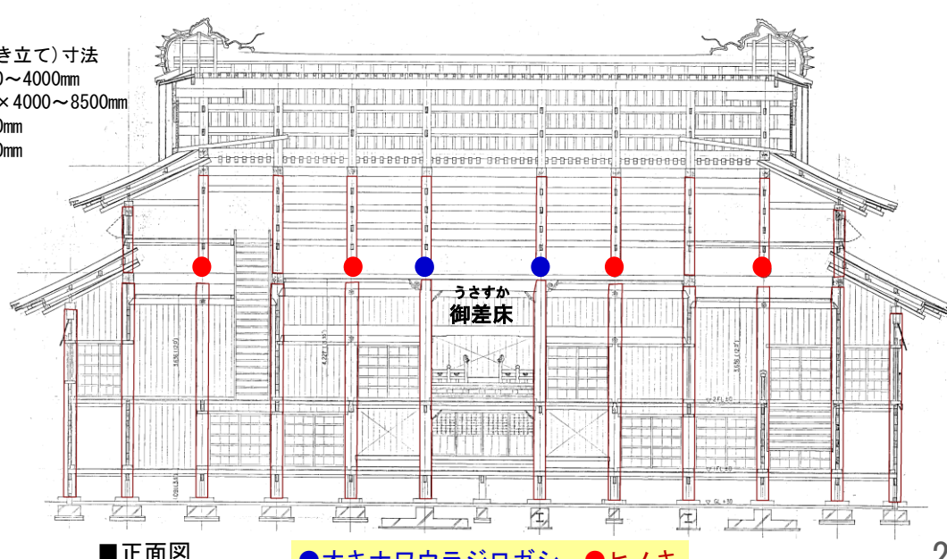
■正面図
