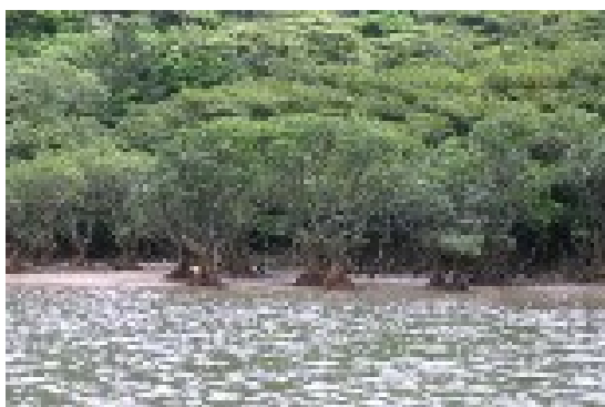
メヒルギ
