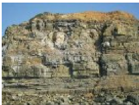
断層の写真
