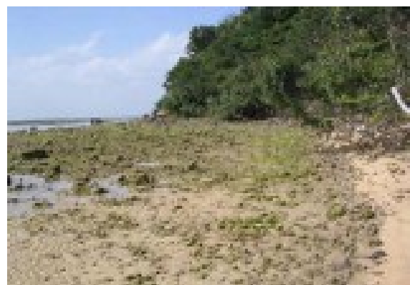
岩礁海岸
