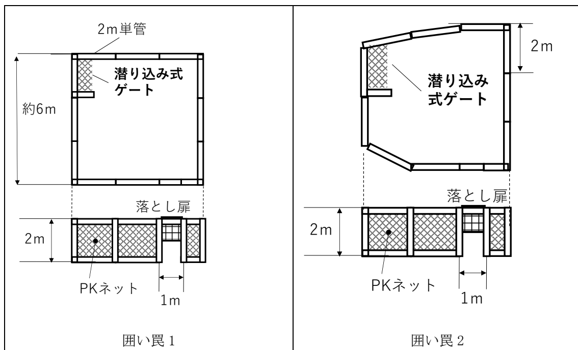
図4 罠の形状
