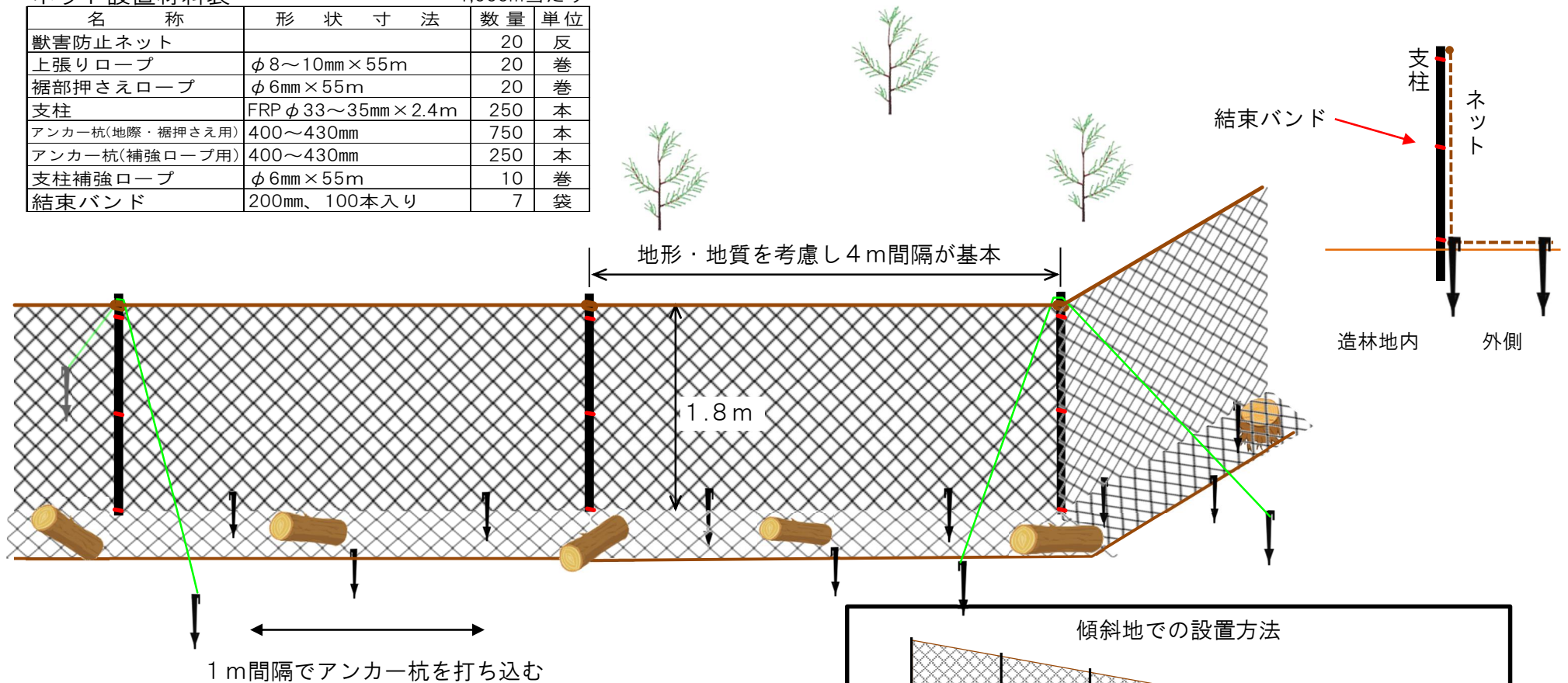
ネット設置材料表
