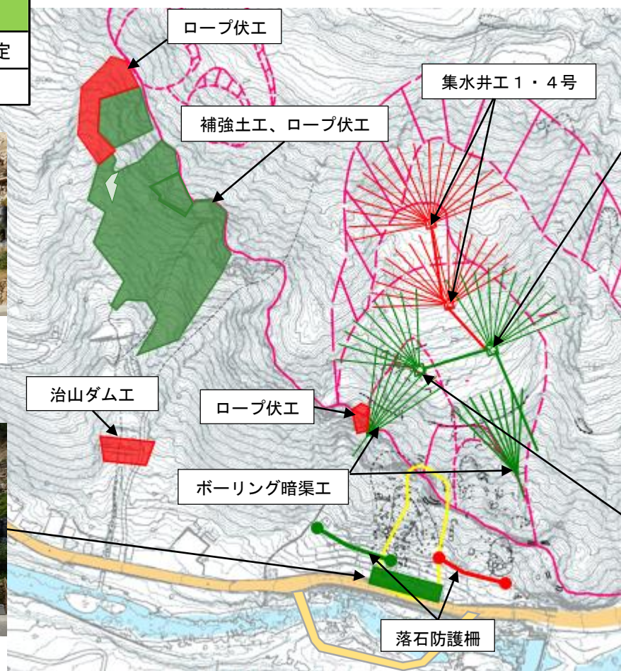
仮設防護柵（幅36m、高さ4m） R1. 11. 13完成
