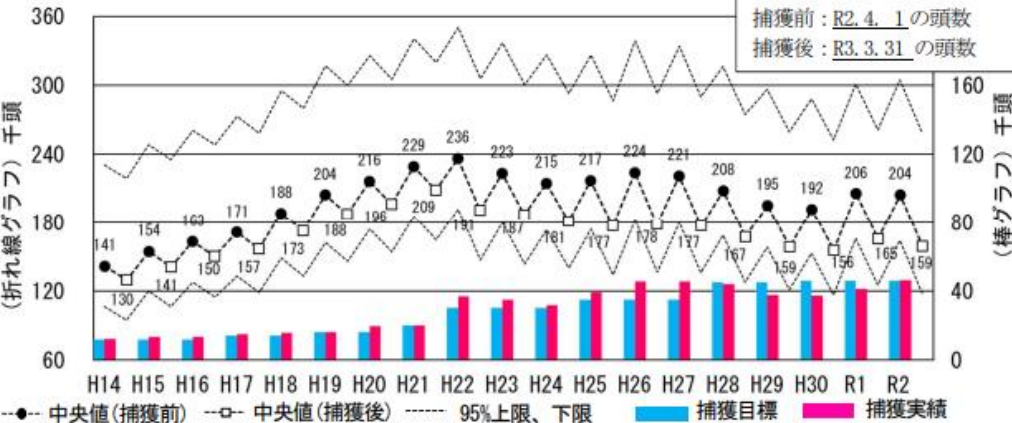
図-1 推定生息数の推移 注：年度内増減は捕獲前と捕獲後の差
