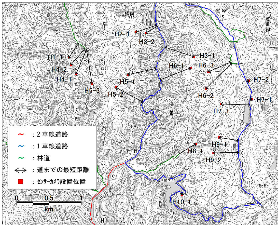
図 4-5 センサーカメラ位置から道路までの最短距離
