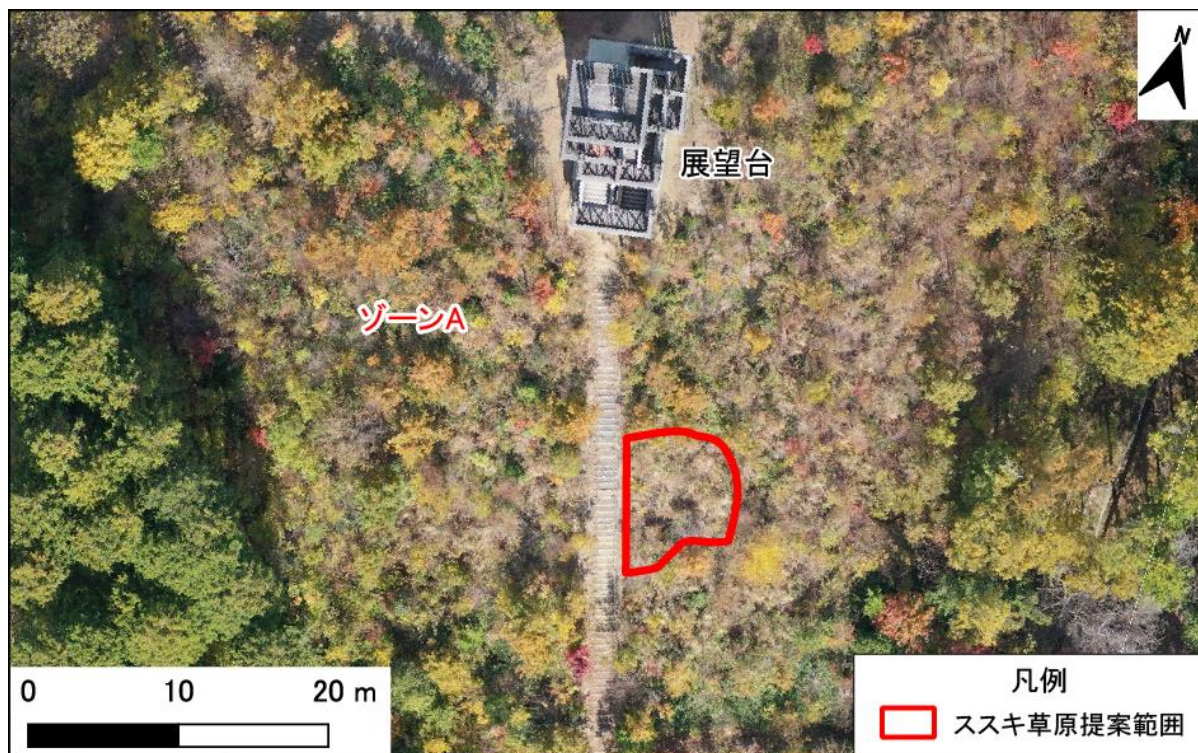
図 7 ススキ草原育成提案範囲
