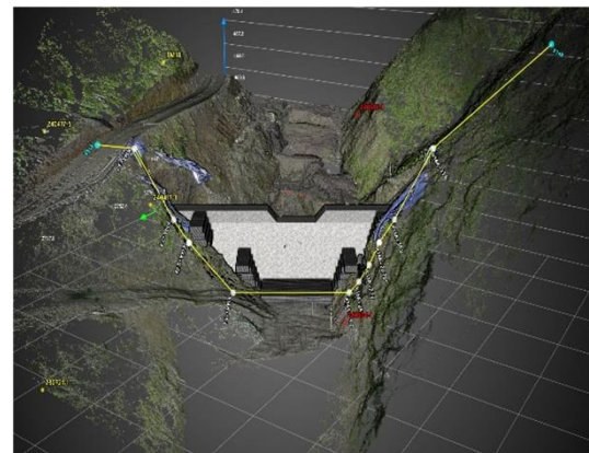
溪間工事の3次元モデルと地形データ (若狭町:河内(こうち)溪間工事)
