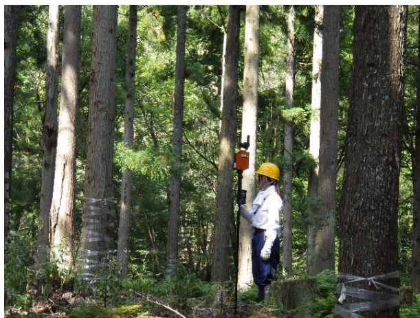
3次元地上レーザスキャナ(OWL)の研修会 (敦賀市:黒河山(くろこやま)国有林)
