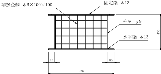
部材リスト（K08型）
