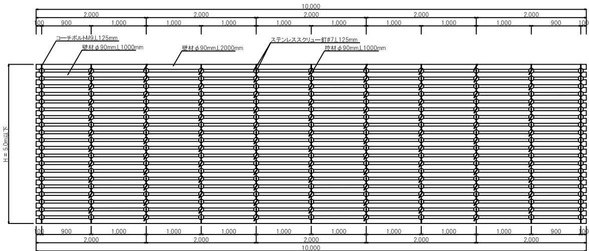
正面（展開）図
