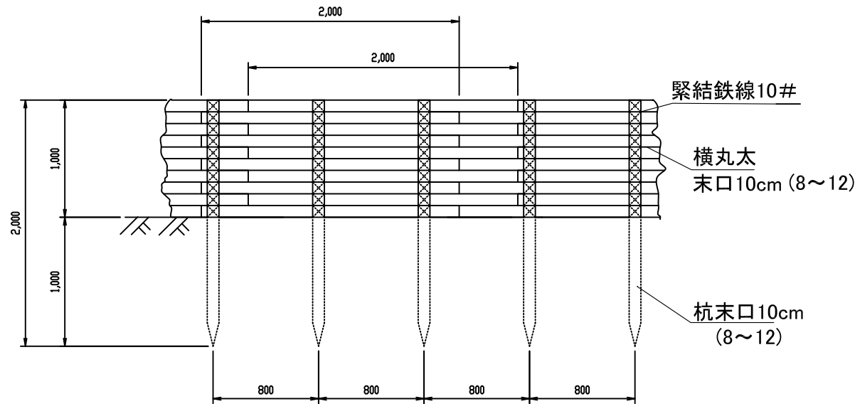
正面図
