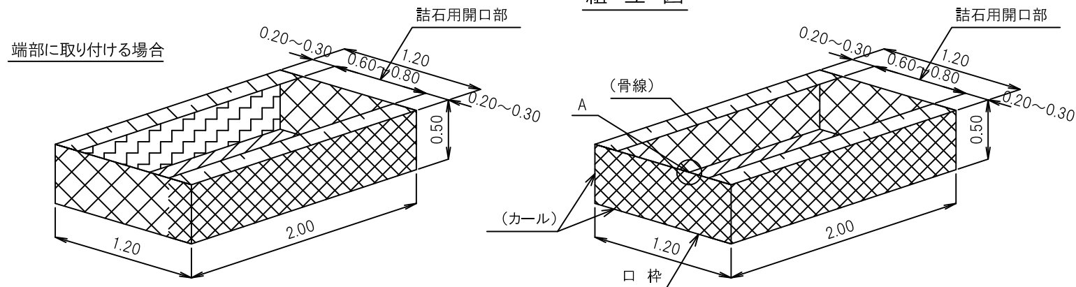
組立図
