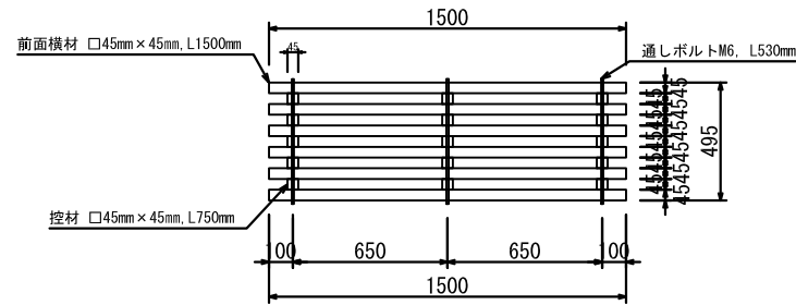
背 面 図
