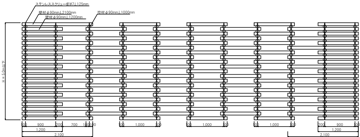
背面（展開）図
