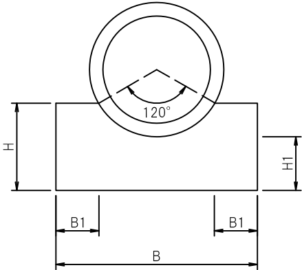
コンクリート基礎 120°
