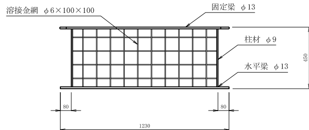
部材リスト（K12型）
