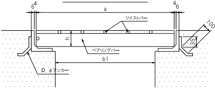
グレーチング断面図
