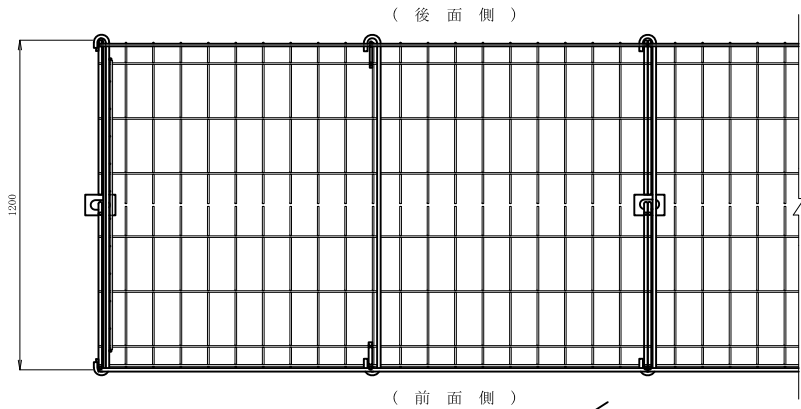
平面図
