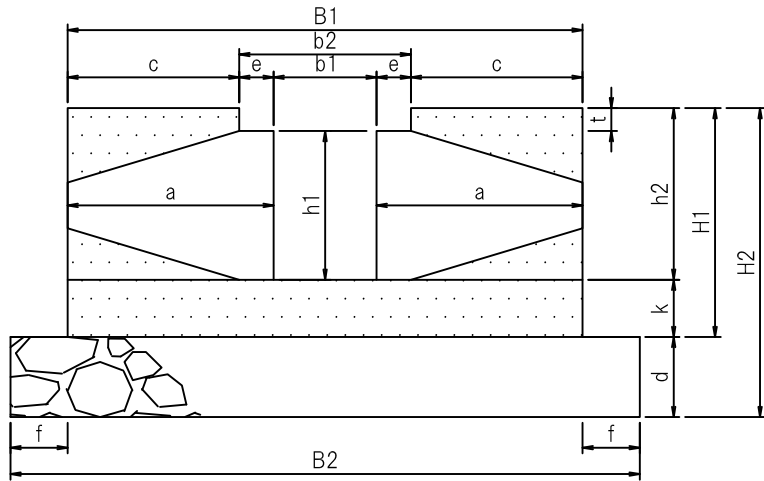
グレーチング横断溝寸法表
