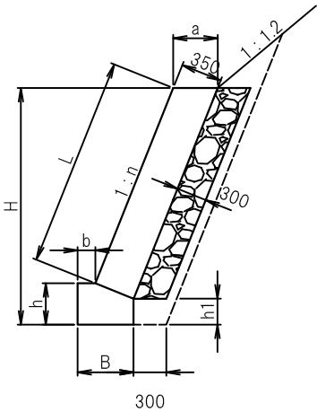
BW-1.2-N-0.3(裏コンなし)
