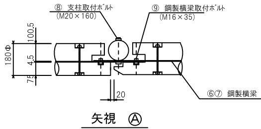
標準設置図
