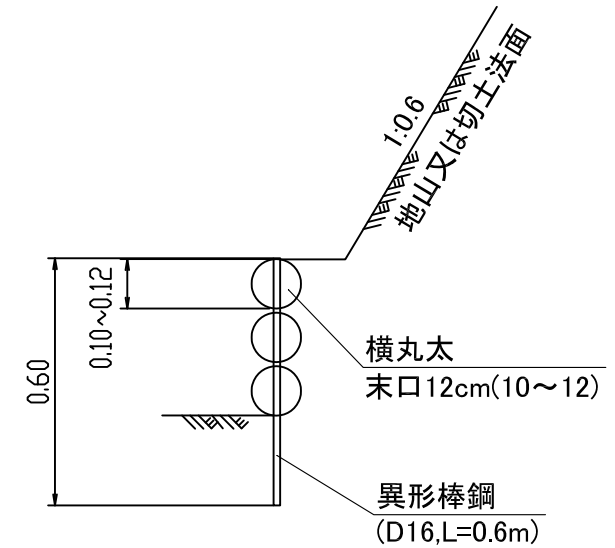
側面図
