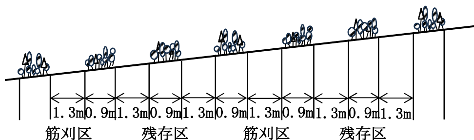
図（側面図）
