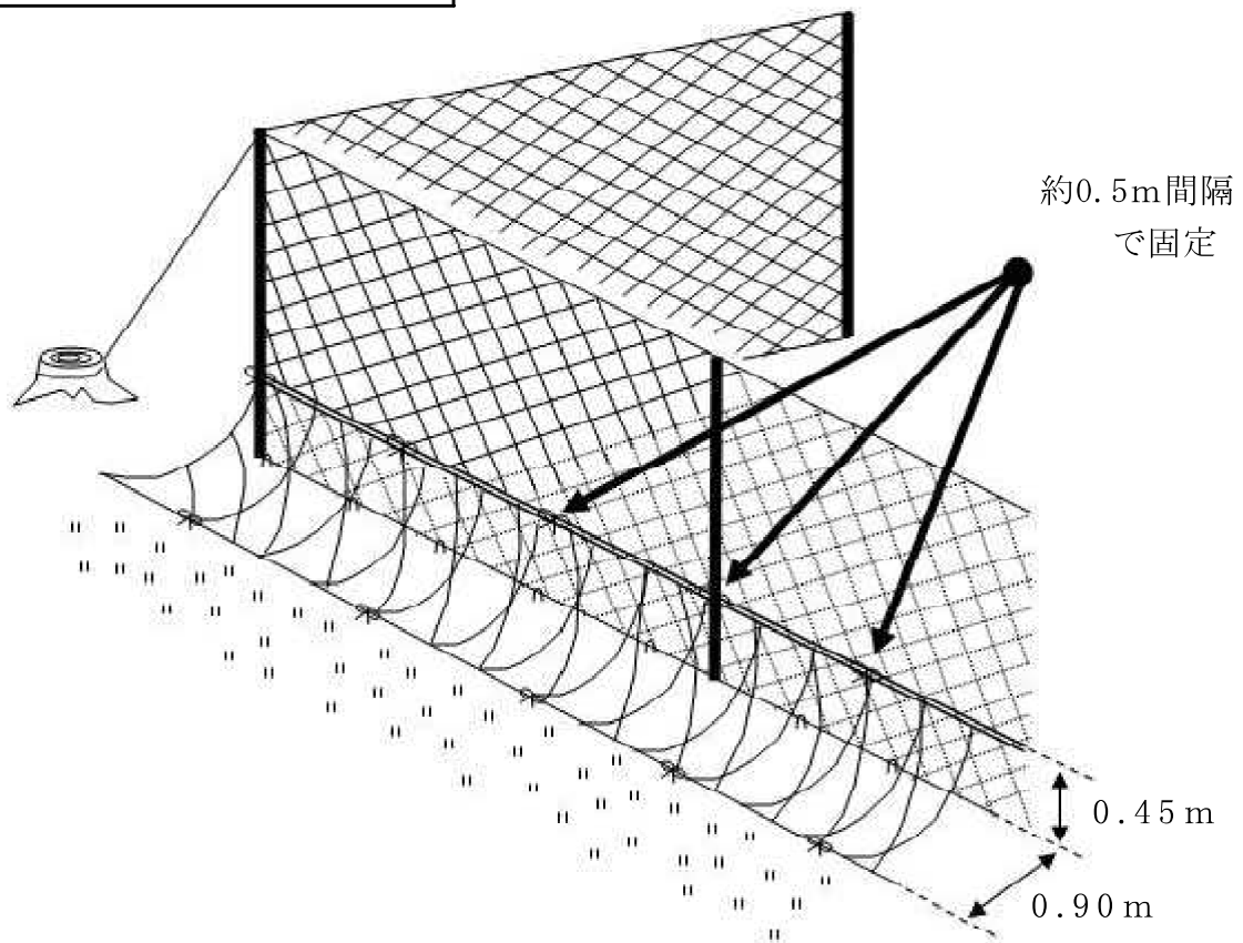
側面図
