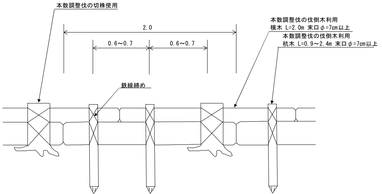
正面図
