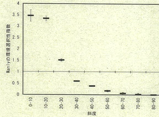
図12 GPSテレメトリー調査による活動点の傾度とその選択性指数
