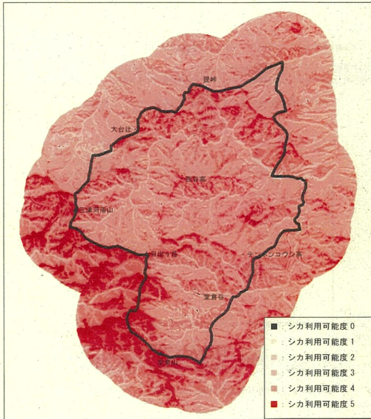
図 15 地形から評価したシカの利用可能度の分布 (□ 調査対象地域) (本事業および環境省公表予定資料を基に作成)
