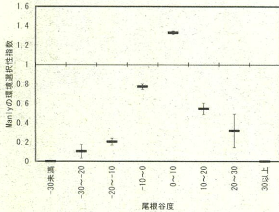
図 14 GPS テレメトリー調査による活動点の尾根谷度階別選択性指数
