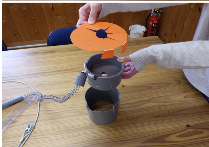
写真2、3 クマ錯誤捕獲を低減させるためのわな （ポリエチレンパイプ製／くくり部径（内パイプ外径）12cm ／上蓋付き／荷重16.5kg／5mmワイヤーセット） ※R7年度は試験的にワイヤー部を既製品ではなく、M・Y式トラップを使用する。
