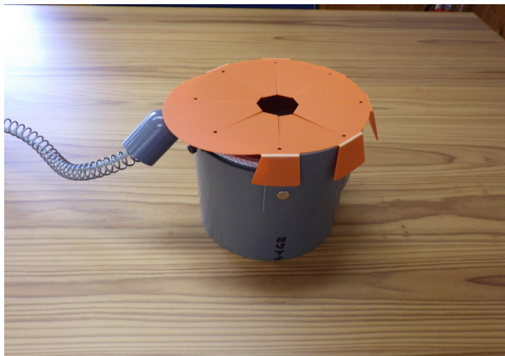
写真1 貸与品（改良型／sサイズ／幅 100mm）
