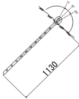
図2-1. イーアンカー打込み角度 岩部用イーアンカー設置角度
