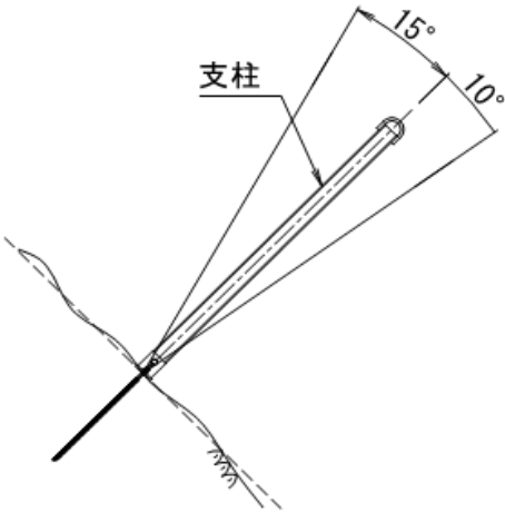
図2-7. 支柱の建込み角度
