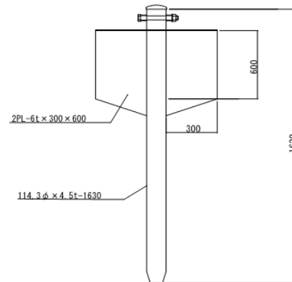
ステーロープ用B型ロケットアンカー
