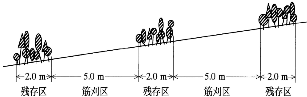
図（側面図）
