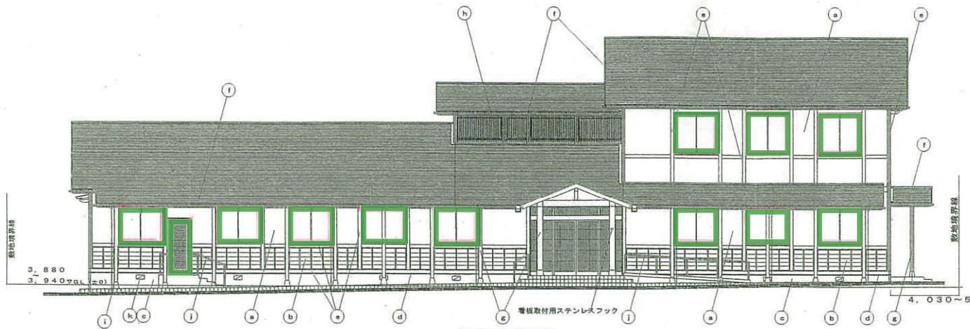
南側立面図
