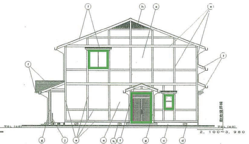
東側立面図
