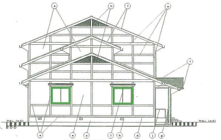
西側立面図
