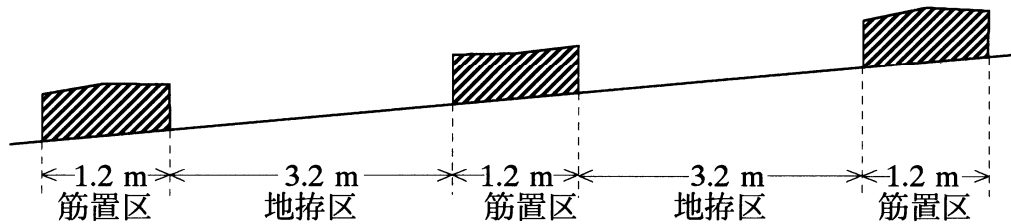
図(側面図)
