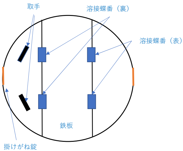
蓋展開図 外径1100mm t3.2mm
